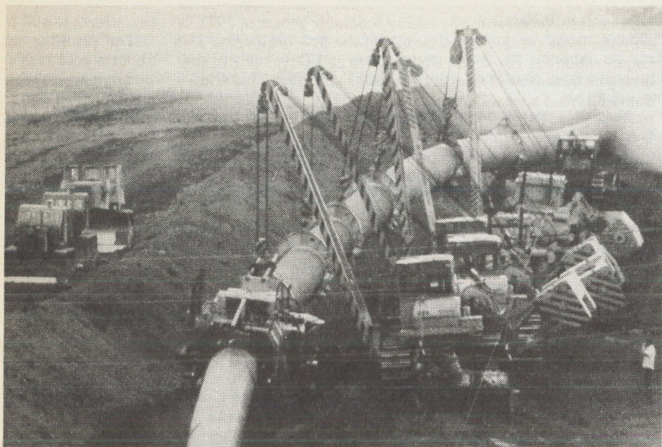
Construction d'un oléoduc en URSS. (DR)
